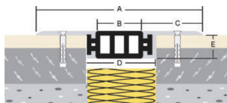
ASM-Profil 230-50
