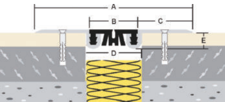
ASM-Profil 240-35
