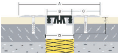
ASM-Profil 241-T-35
