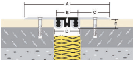
ASM-Profil 240-20
