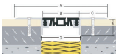
ASM-Profil 241-50
