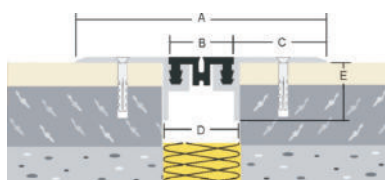
ASM-Profil 241-20
