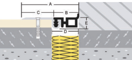
ASM-Profil 240-E
