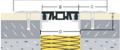
ASM-Profil 241-T-50
