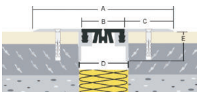
ASM-Profil 241-35
