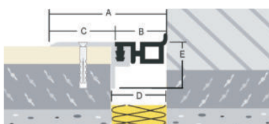
ASM-Profil 241-E
