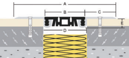
ASM-Profil 240-50
