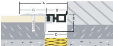
ASM-Profil 241-TE
